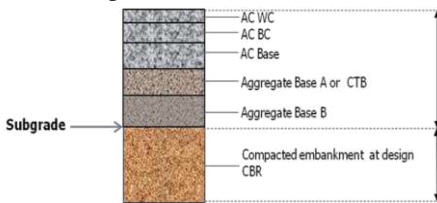
Gambar 2 Perkerasan Lentur Pada Timbunan
