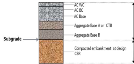
Gambar 1. Perkerasan Lentur Pada Permukaan Tanah Asli (At Grade)
