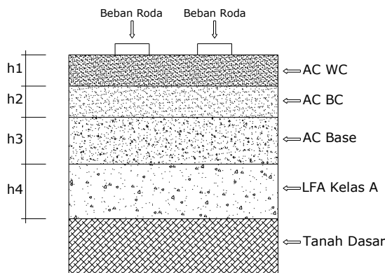
Gambar 5 Tipikal Sistem Perkerasan
