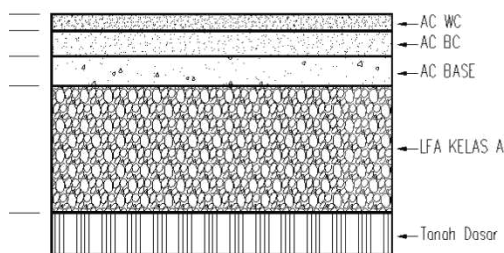
Gambar 8 Susunan lapis prkerasan
