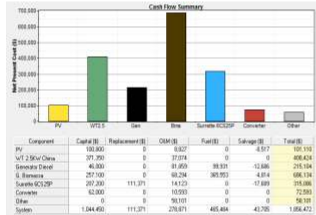
Gambar 15. Ringkasan biaya komponen sistem
