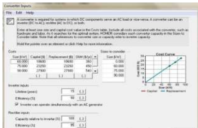
Gambar 10. Parameter masukan bi-directional inverter
