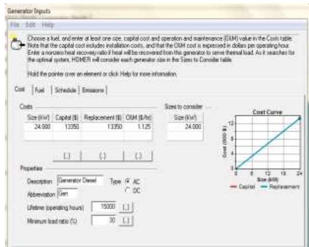
Gambar 9. Parameter masukan generator diesel
