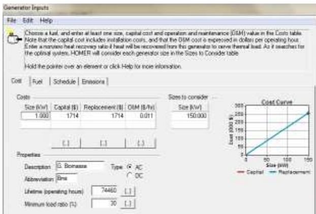
Gambar 8. Parameter masukan gasifikasi biomassa
