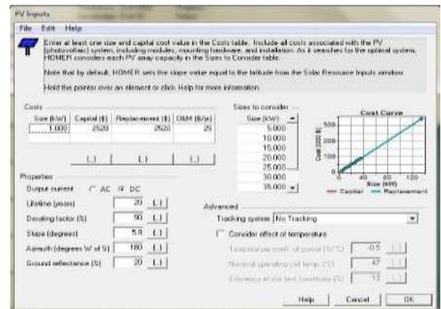
Gambar 6. Parameter masukan panel surya
