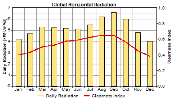
Gambar 3. Potensi energi Matahari di Pulau Nyamuk[10]
