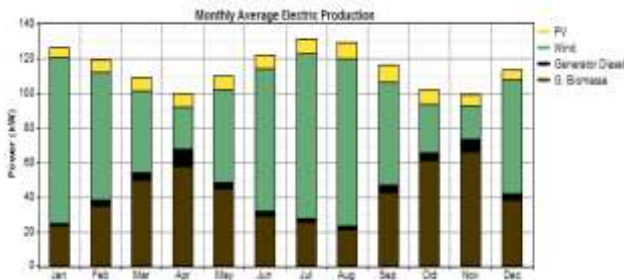
Gambar 14. Produksi energi listrik pada sistem
