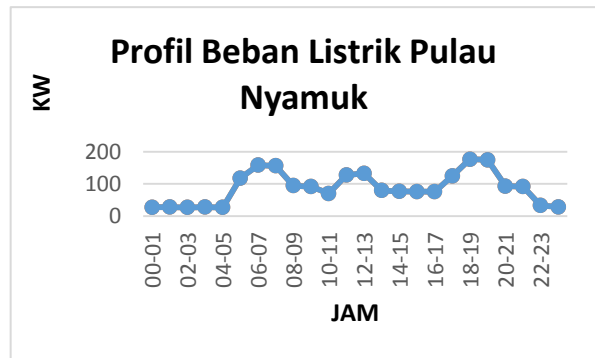
Gambar 2. Profil beban harian Pulau Nyamuk [3]
