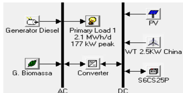
Gambar 12. Konfigurasi sistem pembangkit hibrida saat proses optimasi
