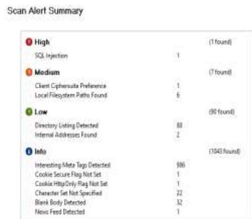
Gambar 7. Hasil scanning oleh vega scanner
