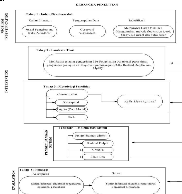
Gambar 2. Kerangka Penelitian
