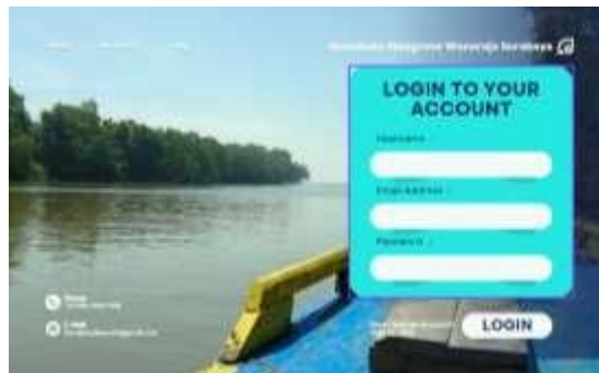
Gambar 2. Halaman Login
