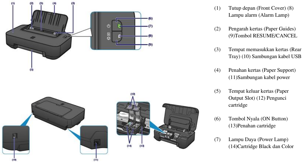
Gambar 3 Komponen-komponen printer
