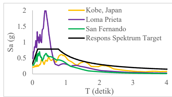
(a) Pseudo-Acceleration tidak terskala arah Y
