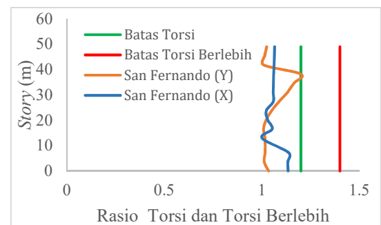
Gambar 10. Ketidakberaturan torsi dan torsi berlebih akibat gempa San Fernando
