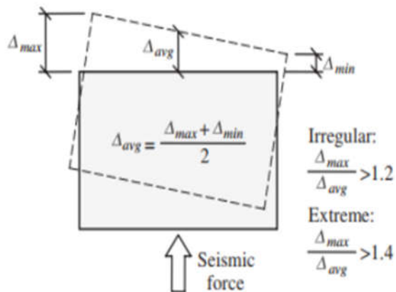
Gambar 7. Ketidakberaturan torsi dan torsi berlebih
